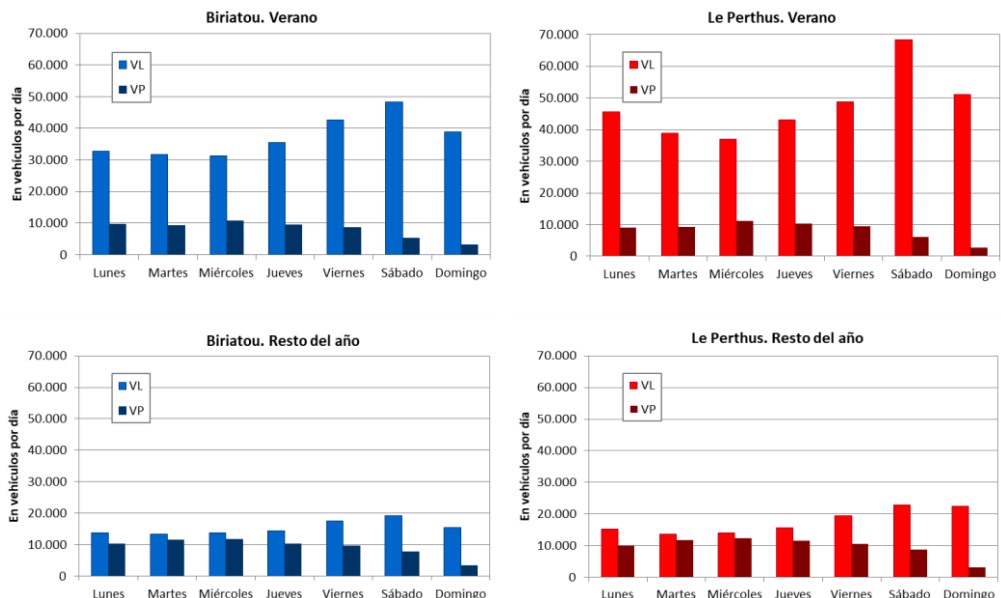
GRÁFICO 14: EVOLUCIÓN DEL TRÁFICO EN LAS AUTOPISTAS LITORALES POR DÍA DE LA SEMANA EN 2015
