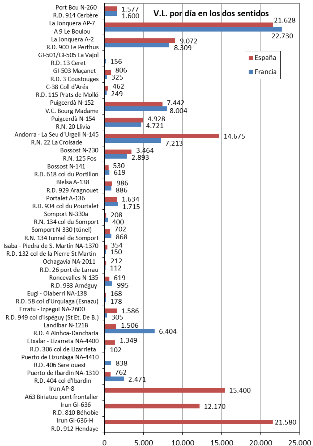
GRÁFICO 17. IMD ANUAL DE VEHÍCULOS LIGEROS EN LOS PASOS FRONTERIZOS EN 2015 (SUMA DE AMBOS SENTIDOS)
