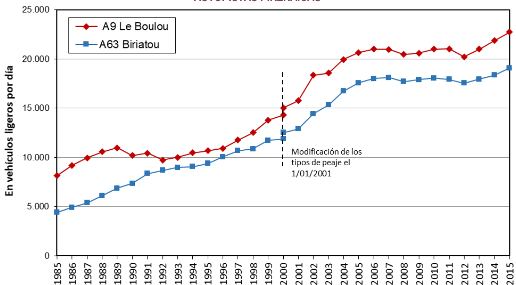
GRÁFICO 19. EVOLUCIÓN DE LA INTENSIDAD MEDIA DIARIA DE VEHÍCULOS LIGEROS EN LAS AUTOPISTAS PIRENAICAS
