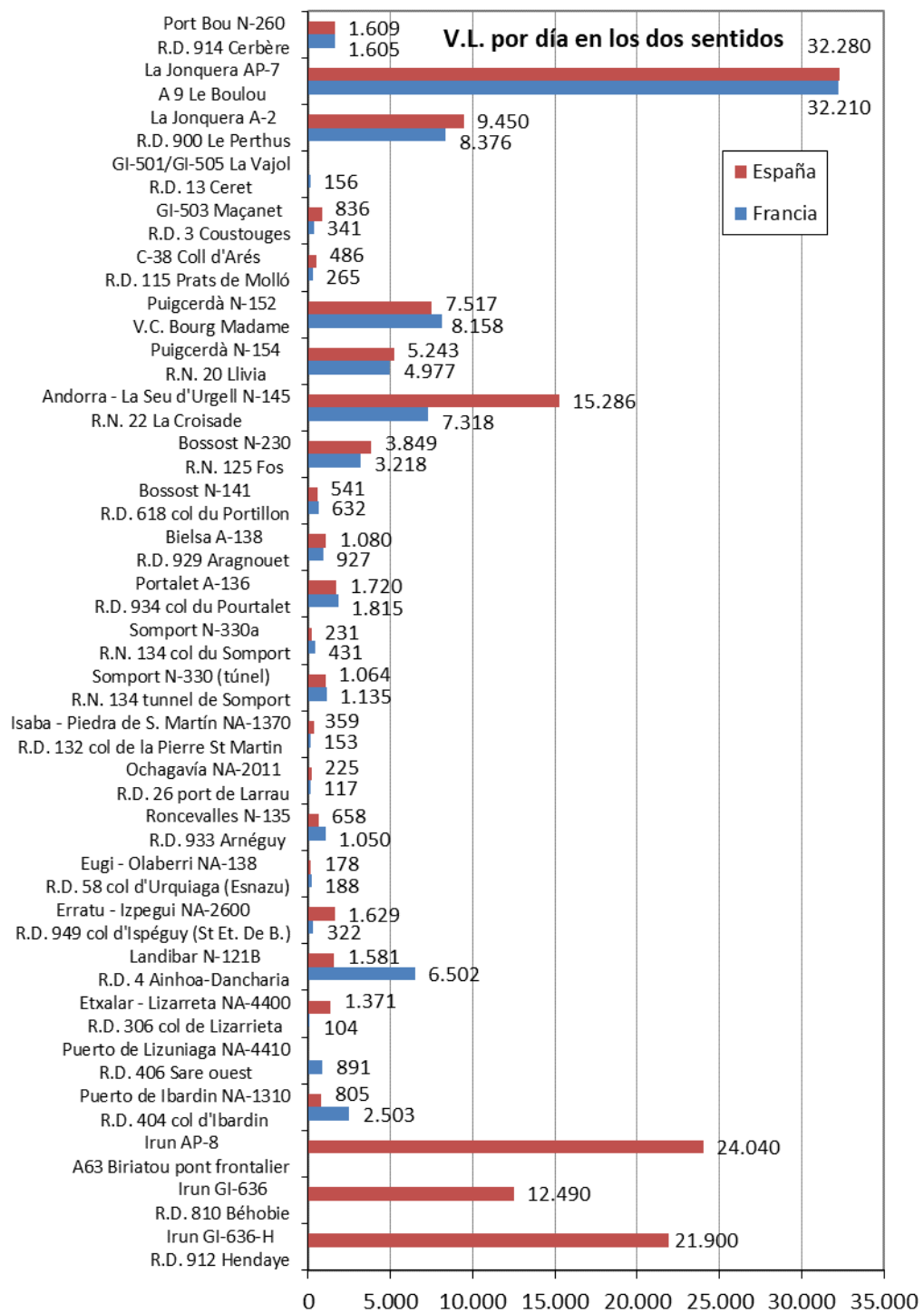
GRÁFICO 11: IMD ANUAL DE LOS PASOS FRONTERIZOS EN EL AÑO 2015 (INCLUIDOS TODOS LOS VEHÍCULOS)
