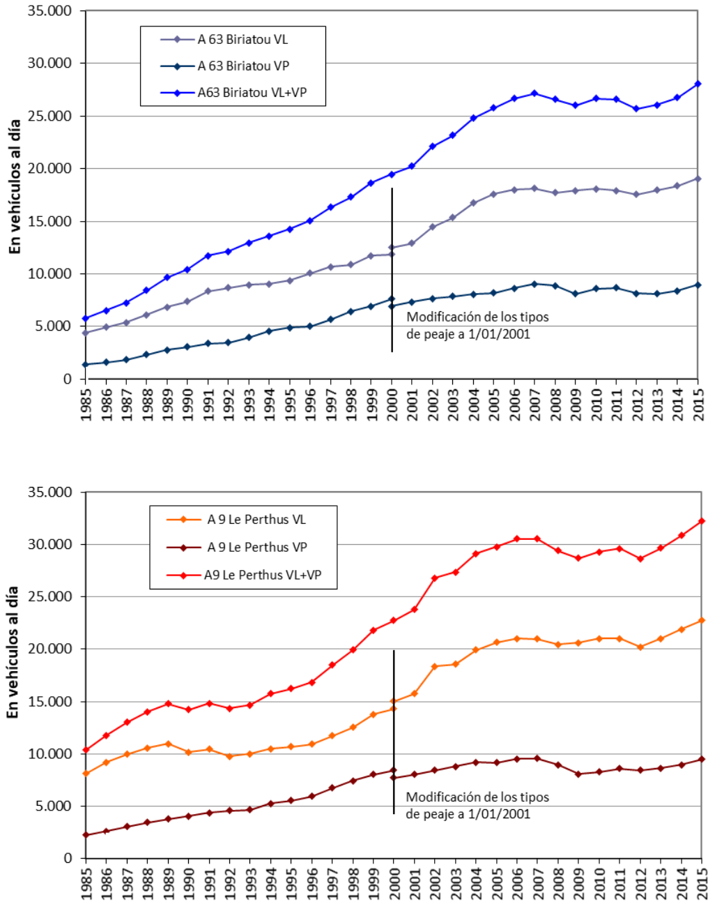
GRÁFICO 16. EVOLUCIÓN DEL TRÁFICO MEDIO ANUAL EN LAS DOS AUTOPISTAS
