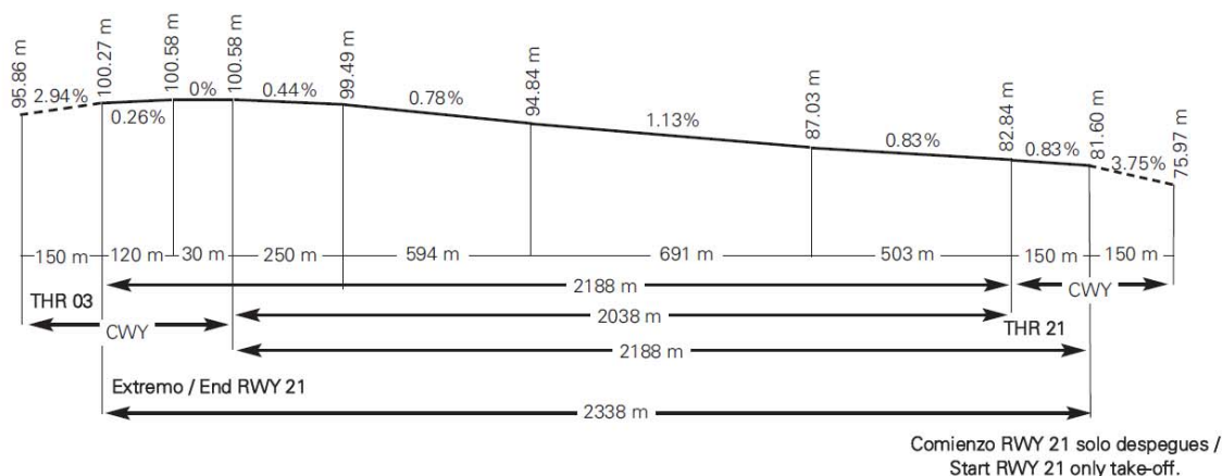
Ilustración 2.3.- Perfil longitudinal de la pista
